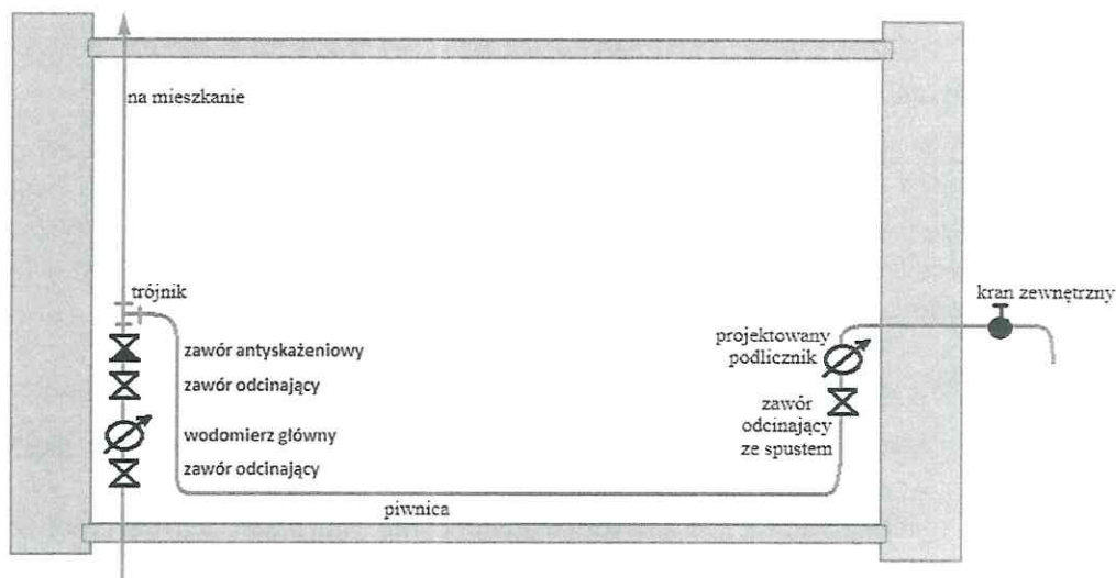
Rys. 1 - Przykładowy schemat ideowy instalacji z wodomierzem ogrodowym (podlicznikiem).
