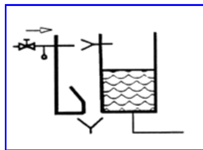
Rysunek A.15 - Zespół zabezpieczający - Symbol graficzny
