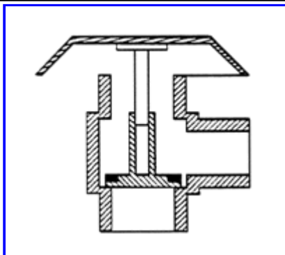
Rysunek A.33 - Urządzenie zabezpieczające - Symbol graficzny
