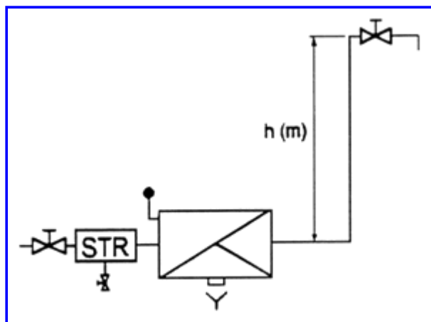
Rysunek A.68 - Instalowanie
