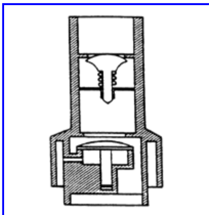
Rysunek A.91 - Konstrukcja
